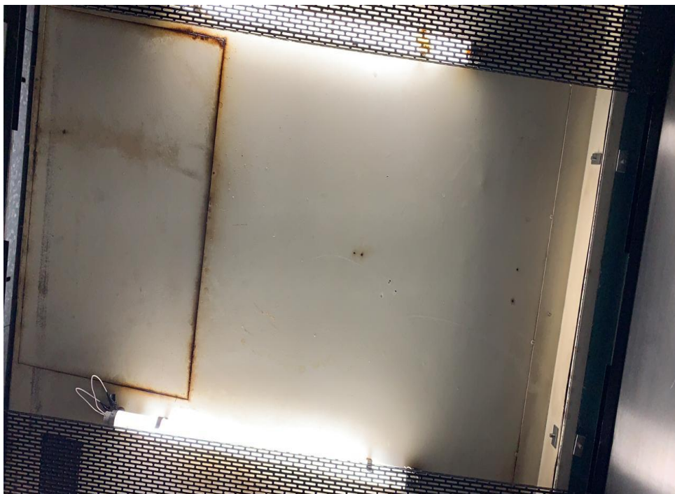
Fig. 4- Adequação do subteto: forro em aço vazado (na imagem apresenta infiltrações por vazamento de óleo), e adequação da iluminação.
