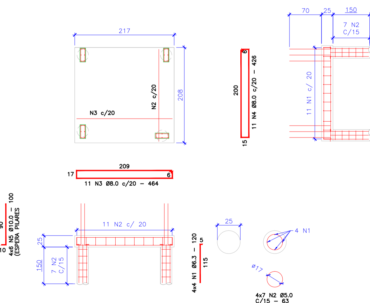
1 DETALHE FERRAGEM FUNDAÇÕES ESCALA: 1:30
